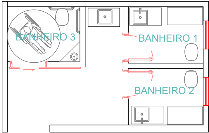
Planta baixa banheiros Sem escala
