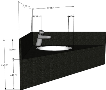
Vista Lateral - Banheiro 3 Sem escala
