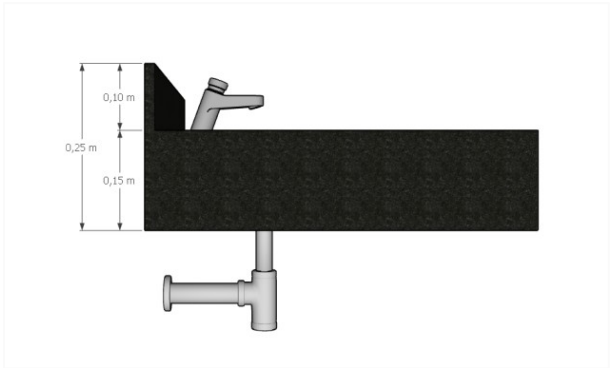
Vista Lateral - Banheiro 1 e 2 Sem escala
